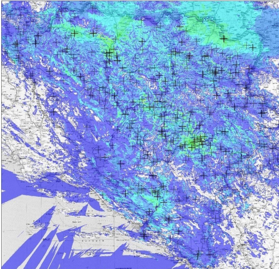
Слика 14. Симултанно покривање аналогних ТВ станица које су још у раду
