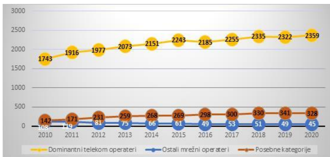
Микроталасни линкови - динамика раста у периоду 2010-2020. за три категорије корисника
